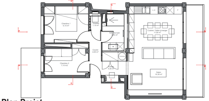
Plan Projet
