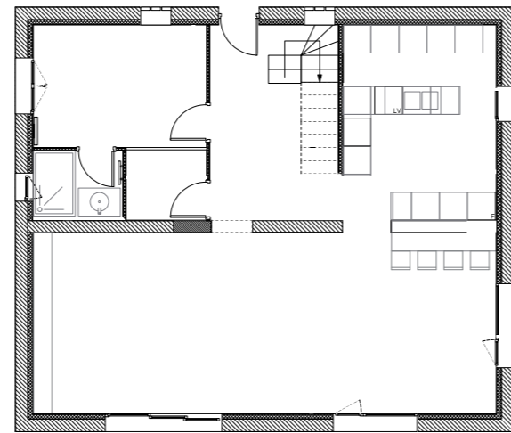
Plan RDC
