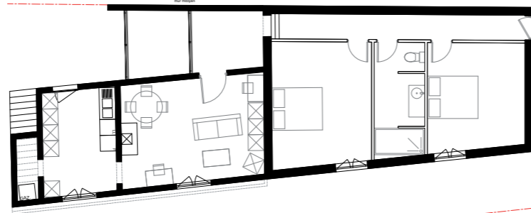
Avant travaux
