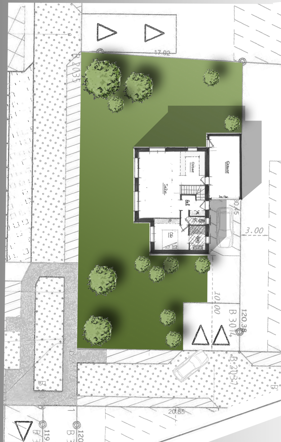
PLAN DE MASSE
