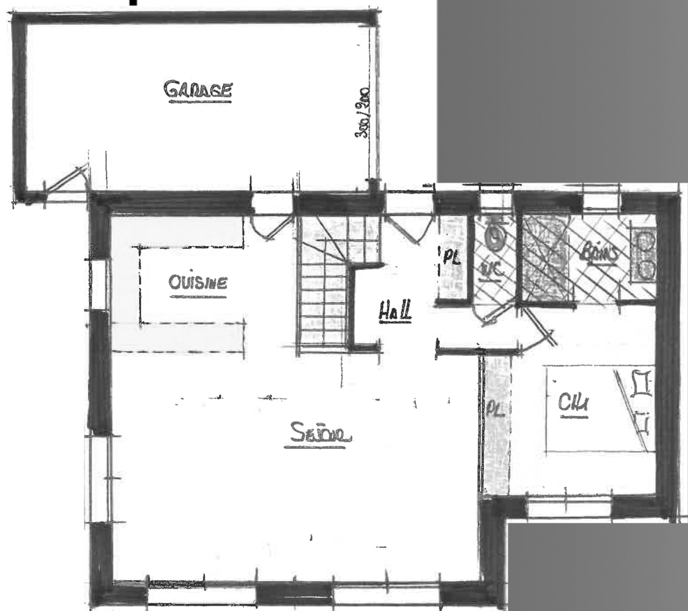
PLAN DE REZ-DE-CHAUSSEE
