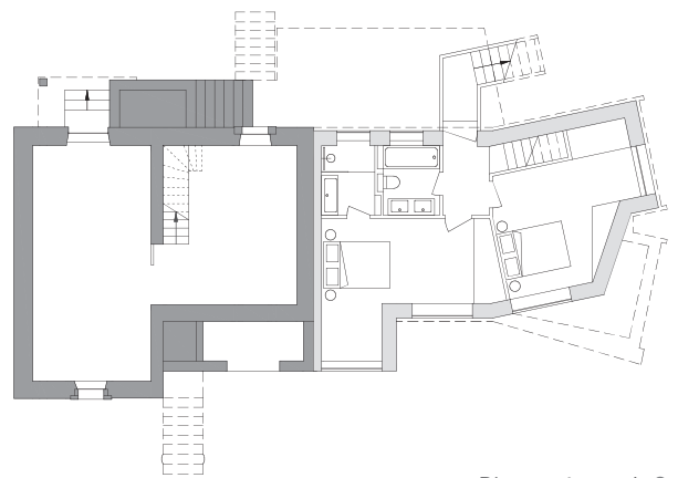
Planta sótano | Cave
