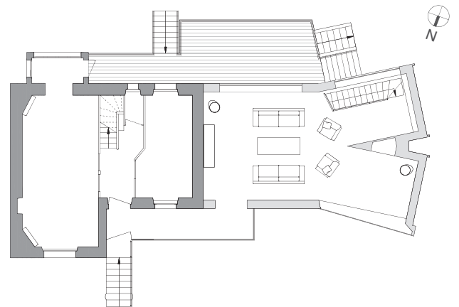
Planta baja | Rez-de-chaussée
