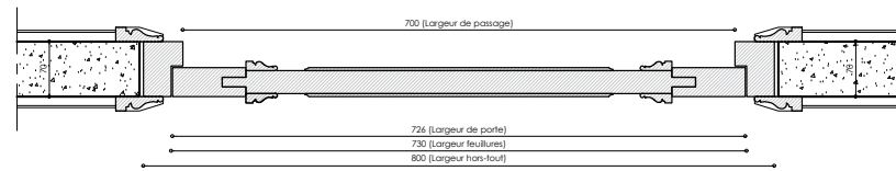
COUPE EN PLAN (grands cadres)
