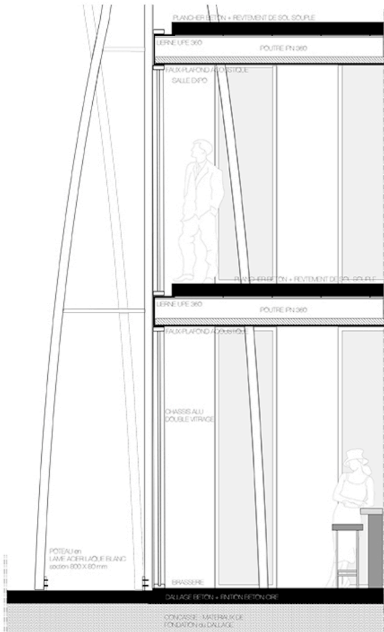
DETAIL ARCHITECTURAL N°1- 1/20° - UN ESPACE PONCTUÉ PAR LA VERTICALITE DES LANIERES STRUCTURELLES CINTREES
