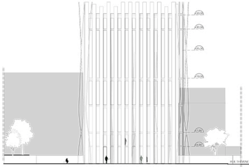
ELEVATION SUD-EST- ech 1/200°
