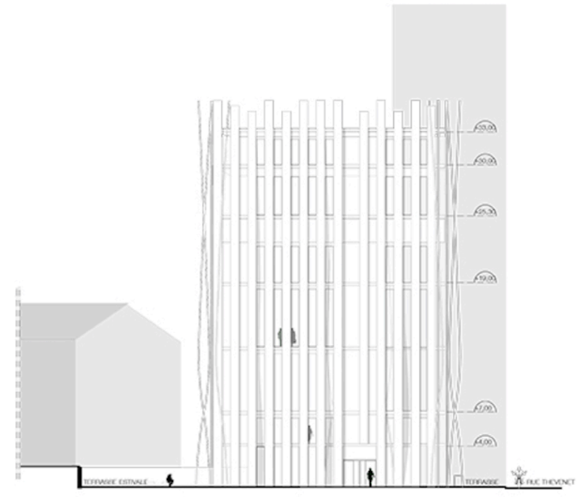
ELEVATION SUD-OUEST- ech : 1/200°
