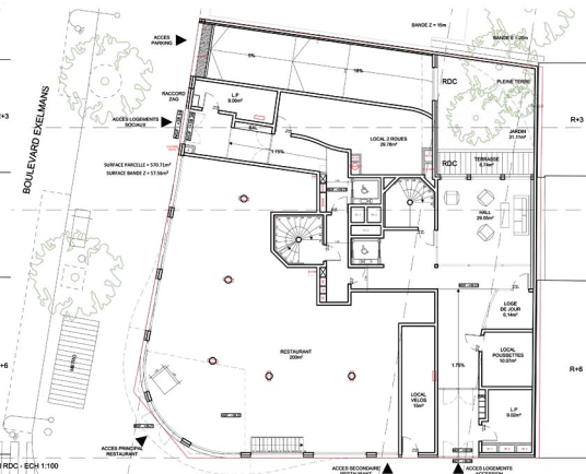
RDC
