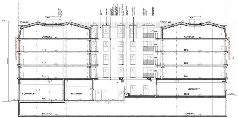
COUPE
