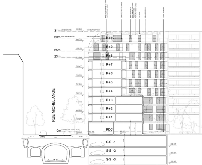
COUPE
