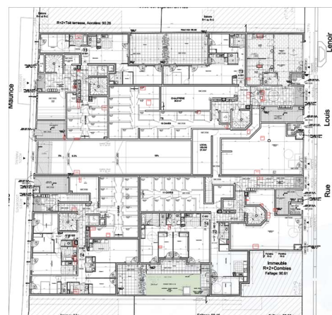
RDC
