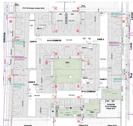
PLAN MASSE
