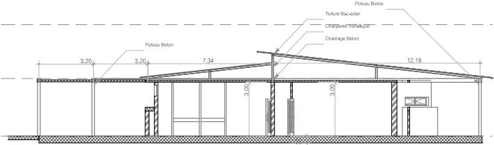
Section de l'auditorium
